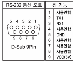
▶ [CN1]
