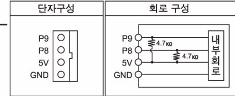
▶ [CN12] CuNET
