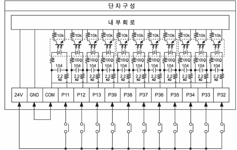
▶ INPUT
