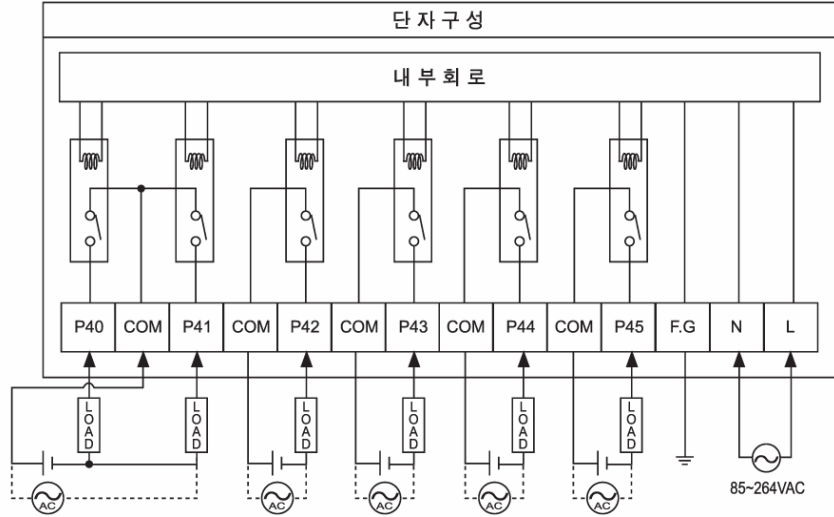
▶ OUTPUT
